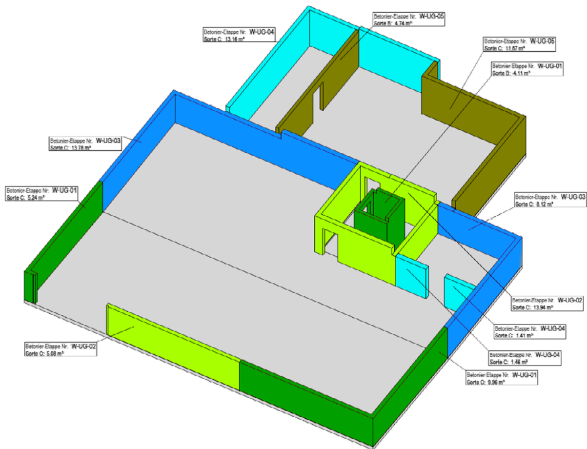
Illustraziun: etappas da betunaziun en in model 3D
